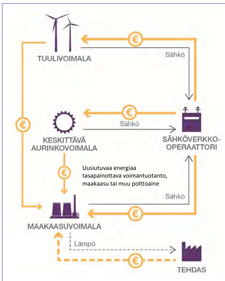
Kuva 20. MetCap Energy'n Karaman, Turkki, voimalaitoksen muodostama energiavirtoja hyödyntävä symbioosi.
